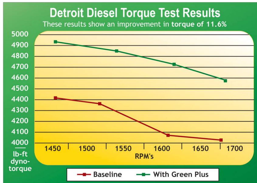
這張圖顯示平均扭力提升11.6%
