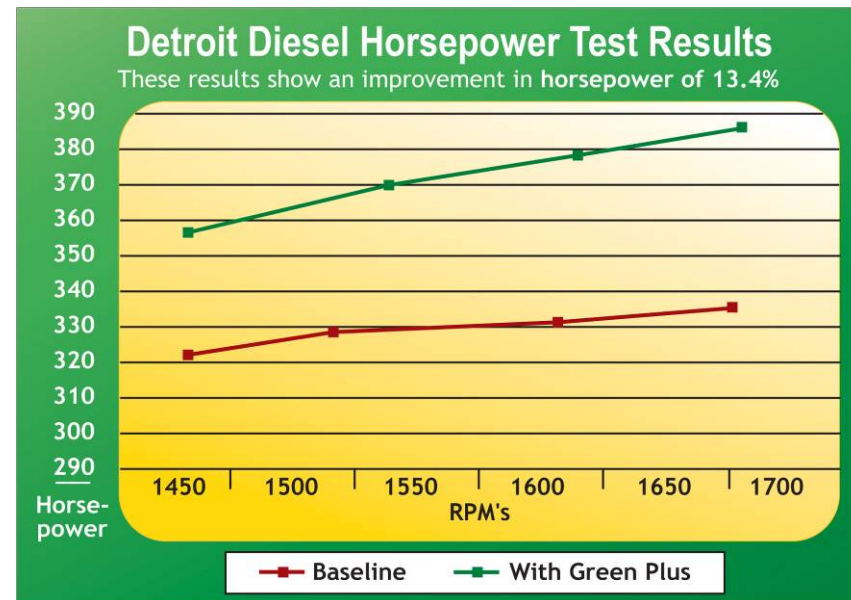
這張圖顯示平均馬力提升13.4%
